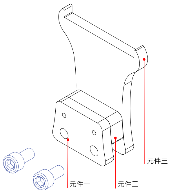
壓克力架組裝圖
